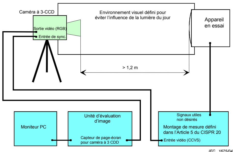
Figure K.1 – Montage de mesure pour évaluation objective de l'image pour un EUT équipé d'un afficheur
